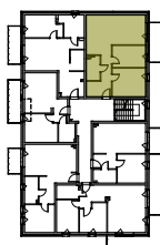
RZUT KONDYGNACJI
